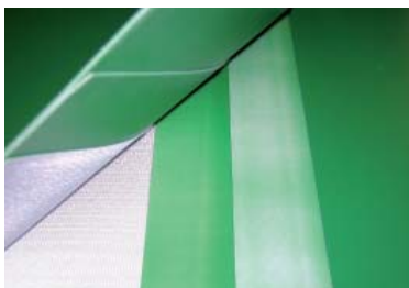
3-lagige Stufenverbindung
