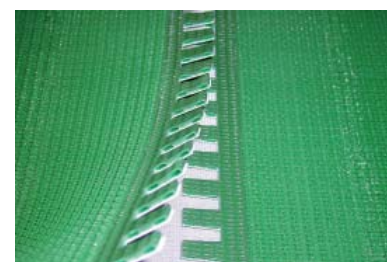
PVC/PU Minet-Verbinder
